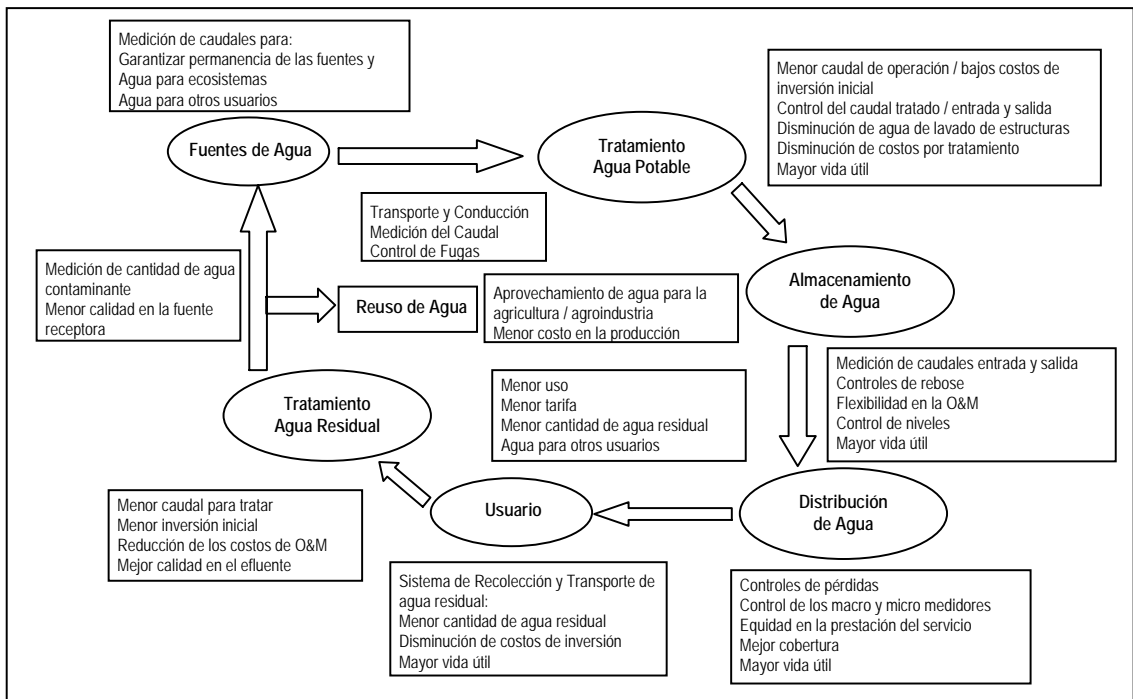
Figura 3. Uso eficiente del agua en el ciclo antrópico
